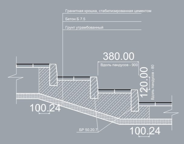
Конструкция лестницы
