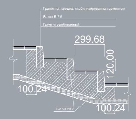
Конструкция лестницы
